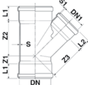
SN8 - SDR34
