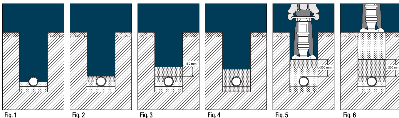
Fig. 1 - Strato di materiale di riempimento compattato a mano fino alla metà del tubo
