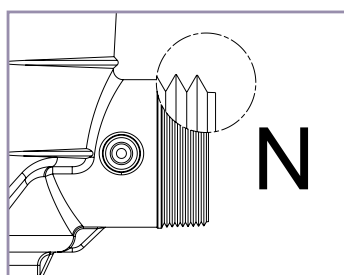
Filettatura NPT
